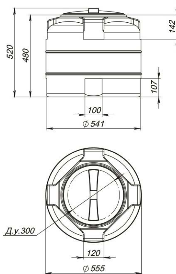
Габаритные размеры ёмкости
