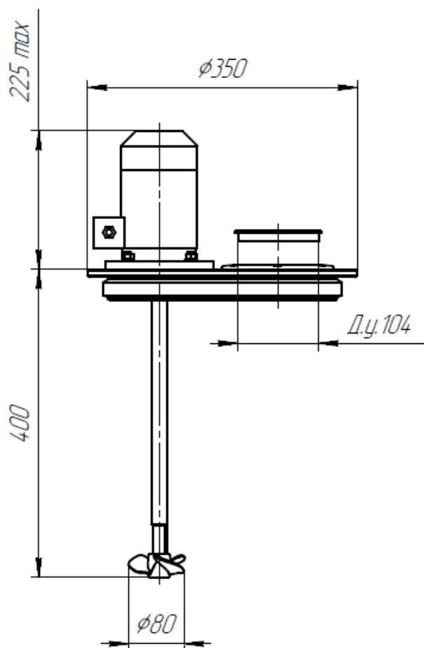
Габаритные размеры миксера
